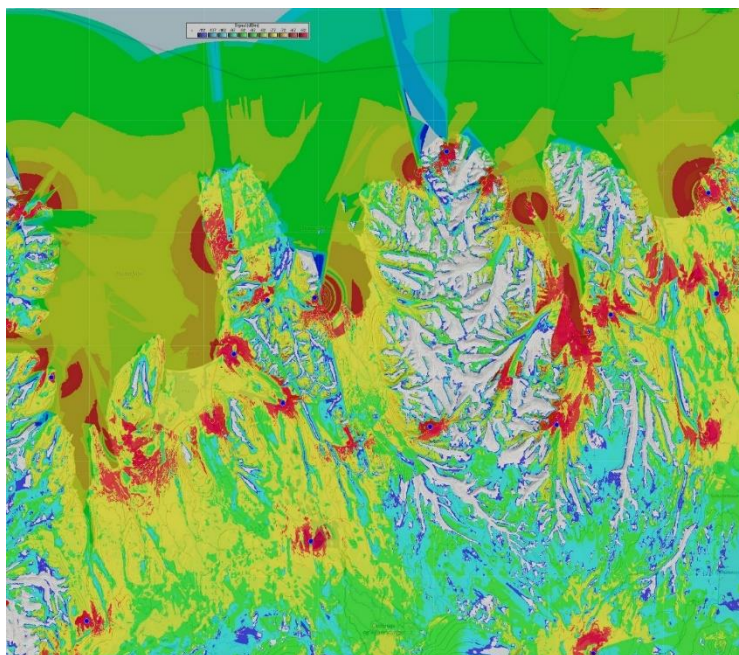
Mynd 14. Tetrasamband á Norðurlandi vestra, 3W bílstöð, 0 db loftnet í 2m hæð mv. 90% tilfella. Litur merkir miklar líkur á þjónustu en þar sem er ólitað/hvítt er ólíklegt að sé þjónusta eða hún gloppótt. Dökkblár litur er dekkun á mörkunum. Mynd, Neyðarlínan.
